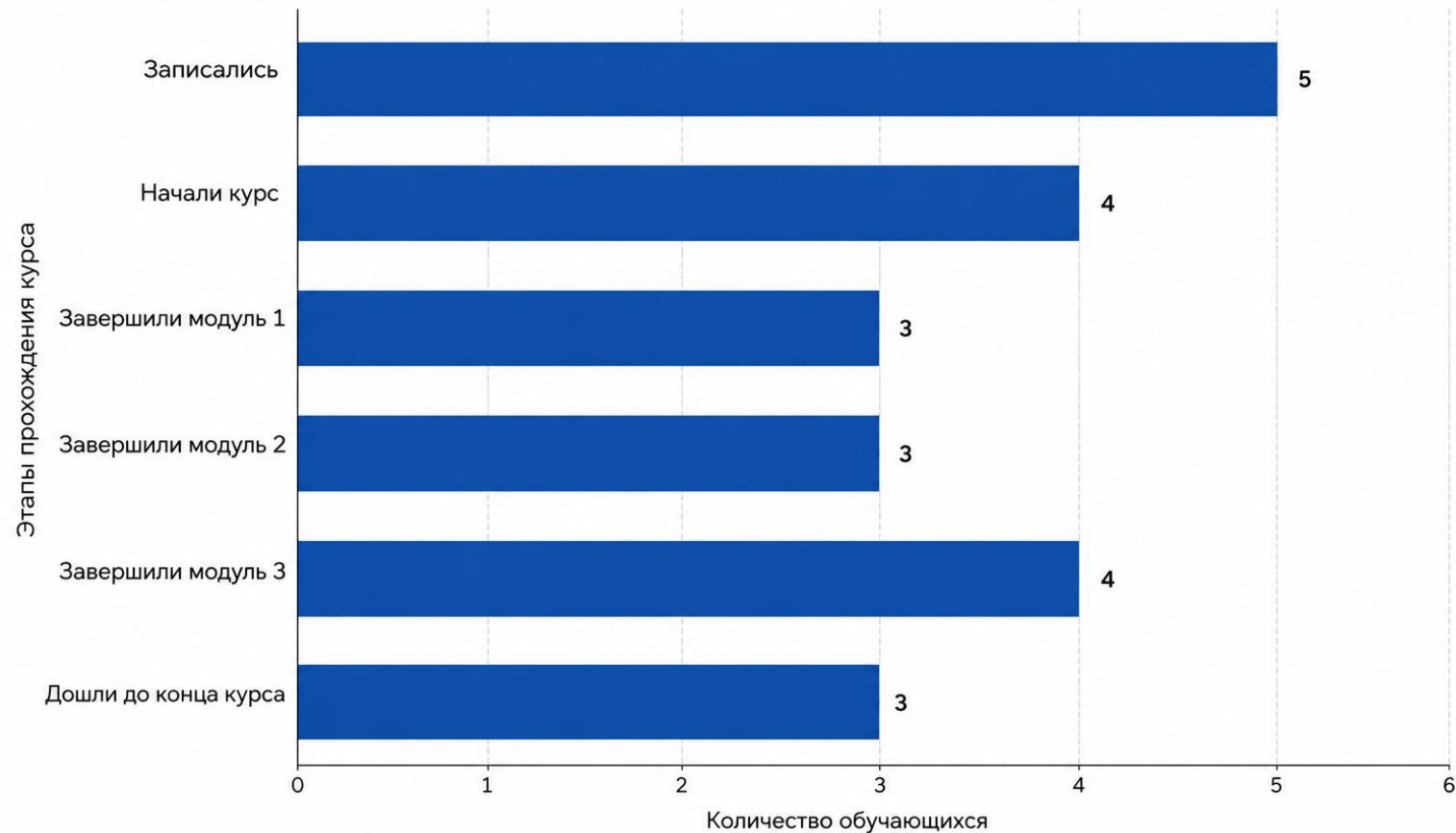
Рисунок 3 — Воронка обучения
